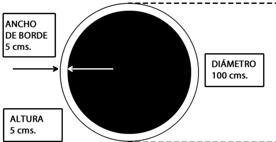
Figura 1. Especificaciones Dohyo
