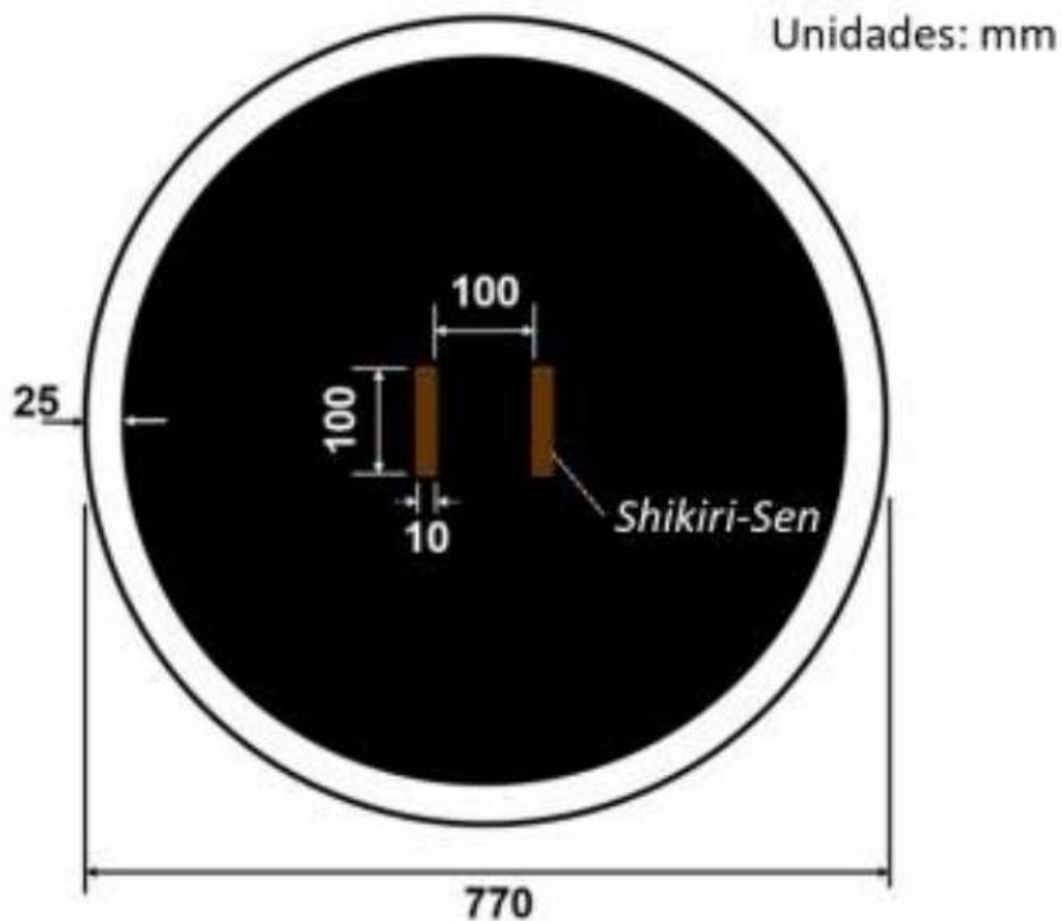
Figura 1. Especificaciones dohyo
